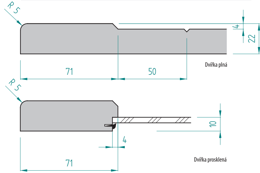
Provedení dvířek D32
