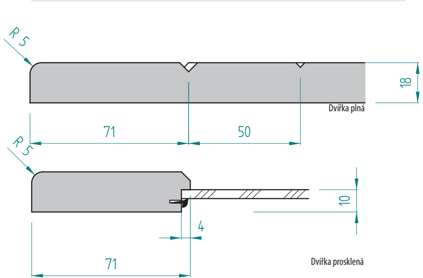
Provedení dvířek D33
