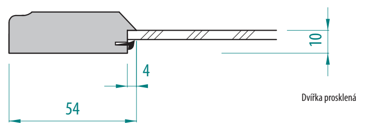
Provedení dvířek D15
