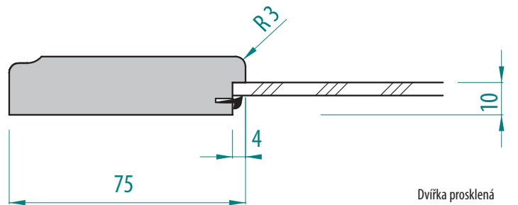
Provedení dvířek D09
