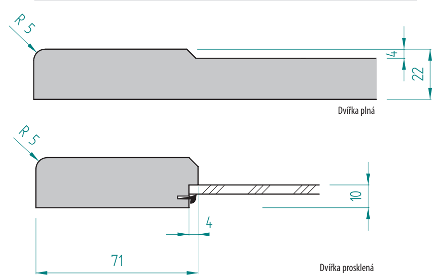
Technické nákresy
