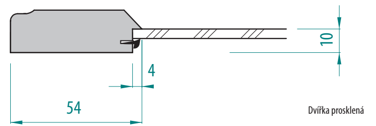
Provedení dvířek D16
