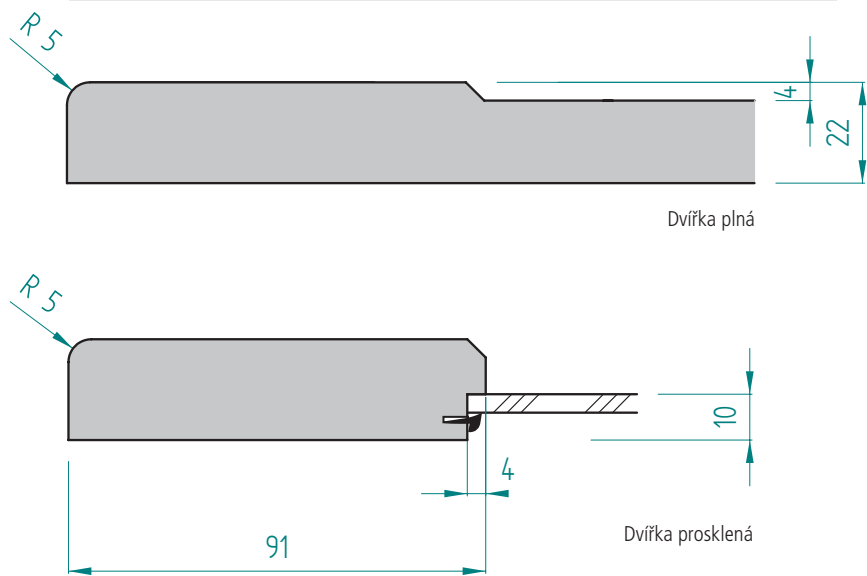
Provedení dvířek D08
