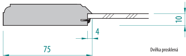
Provedení dvířek D05
