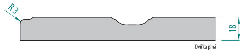
Technické nákresy
