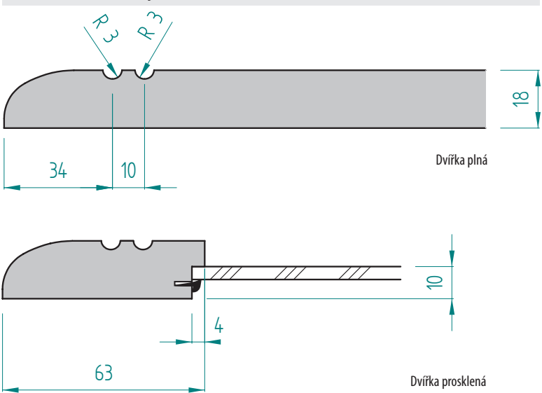
Technické nákresy
