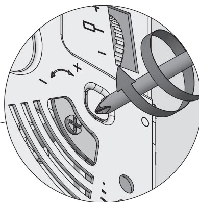
regulace síly otevírání
