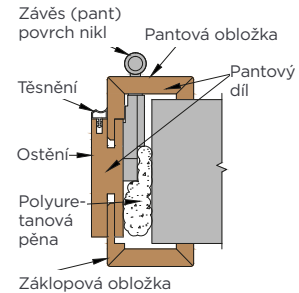
Zárubeň se spojem na pokos
