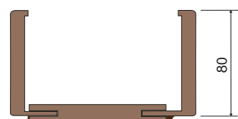
profil zárubně č. 2
